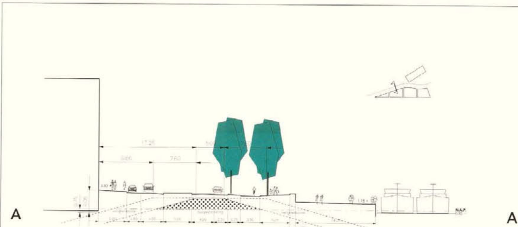
Doorsnede A-A
